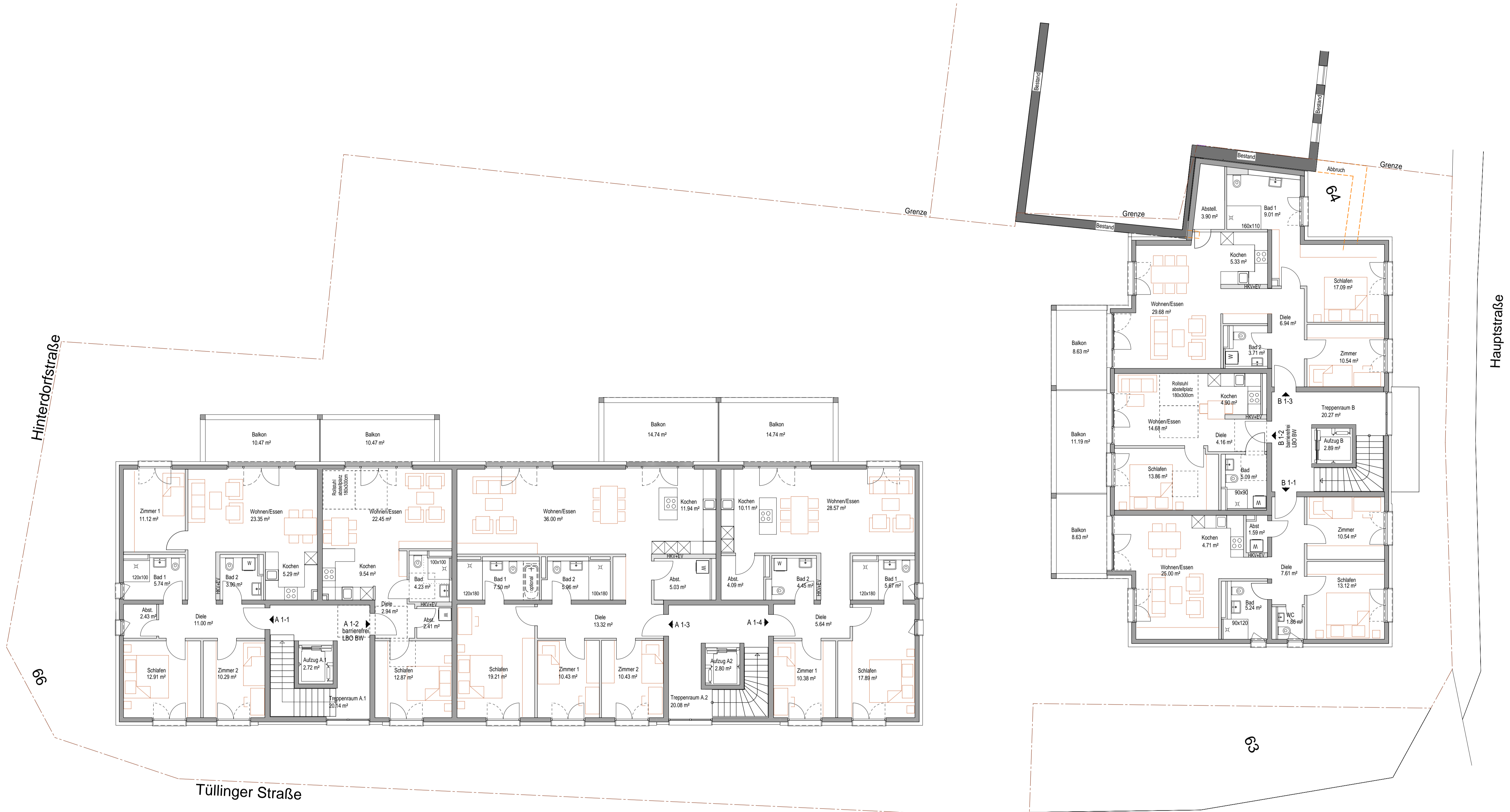
OBERGESCHOSS M. 1:100
